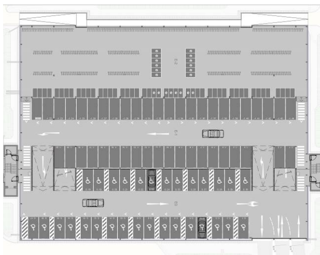
Grundriss Regelgeschoss
