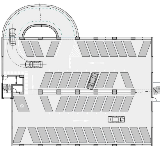
Grundriss Regelgeschoss
