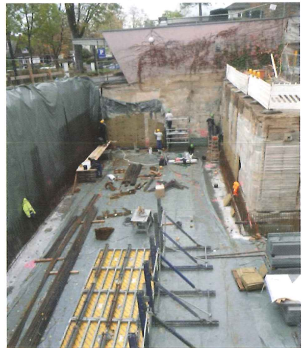
Baustelle nach Betonieren der Bodenplatte
